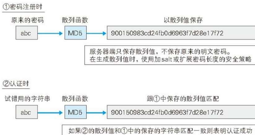
图：破解已加密的密码
