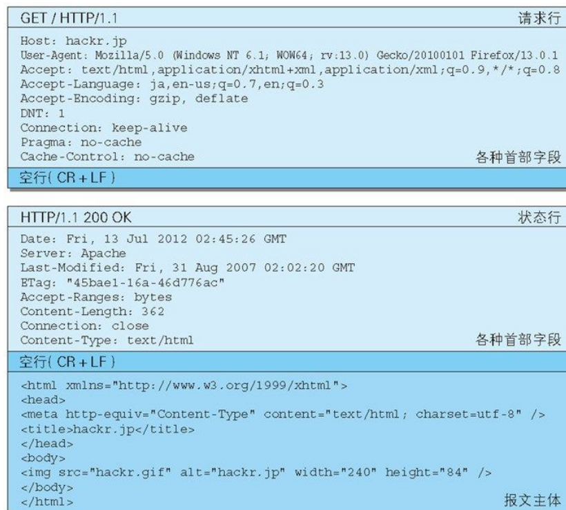
图：请求报文（上）和响应报文（下）的实例
