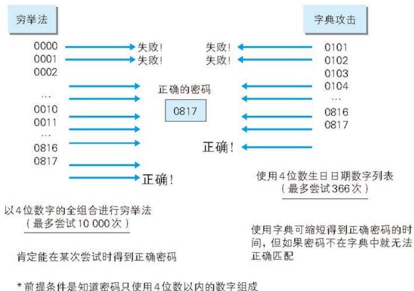
图：穷举法和字典攻击
