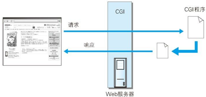
CGI是将请求转给CGI程序处理的一种机制
