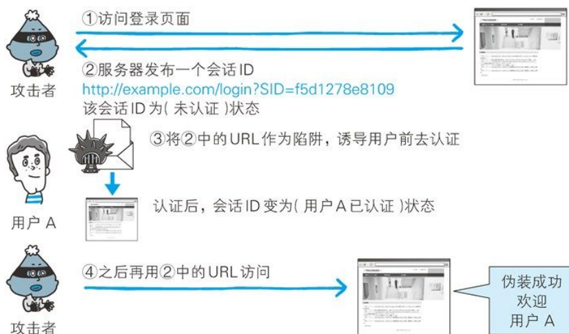
图：会话固定攻击案例
