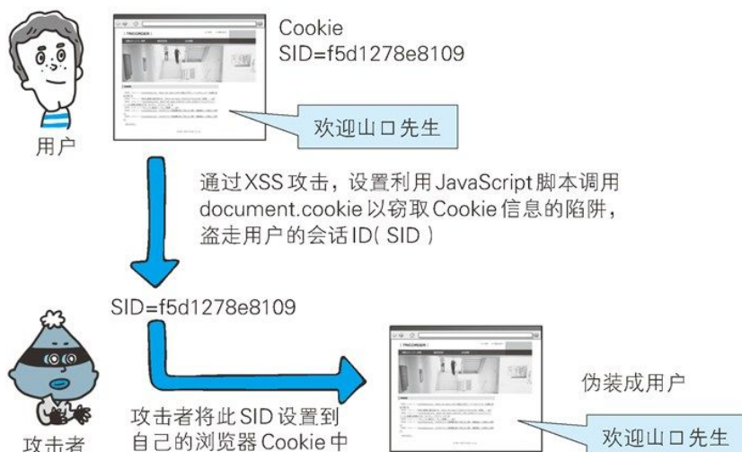
图：会话劫持攻击案例
