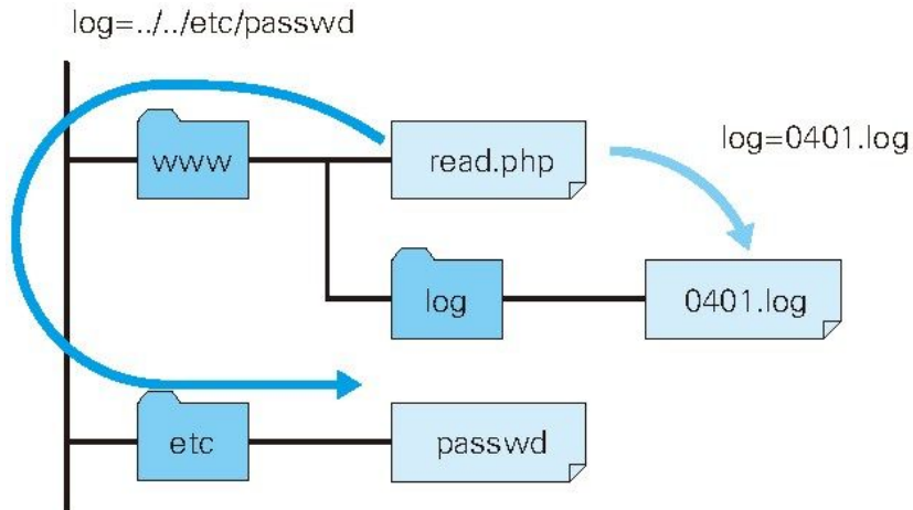
图：目录遍历攻击案例
